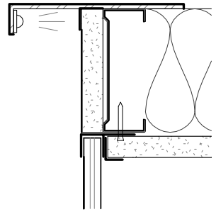
COUPE – VERRE / GYPSE
