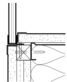
PLAN – VERRE / GYPSE
