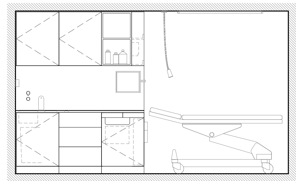
ÉLÉVATION – SALLE D'EXAMEN
