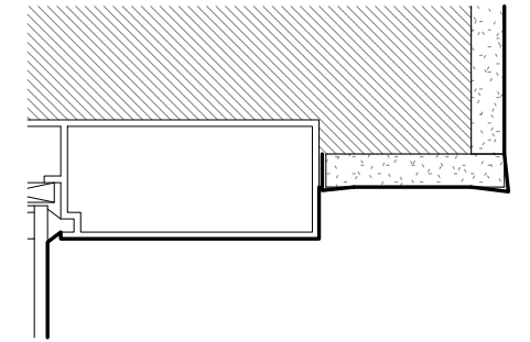
COUPE – LINTEAU FENÊTRE
