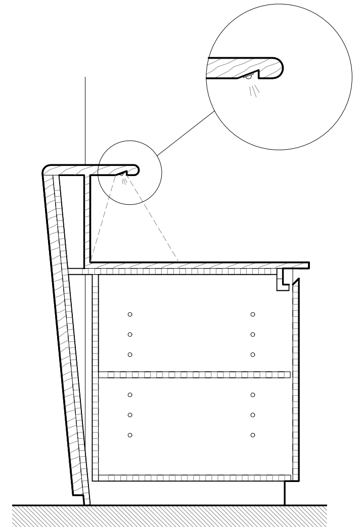
COUPE – ARMOIRE BASSE BUREAU ACCUEIL
