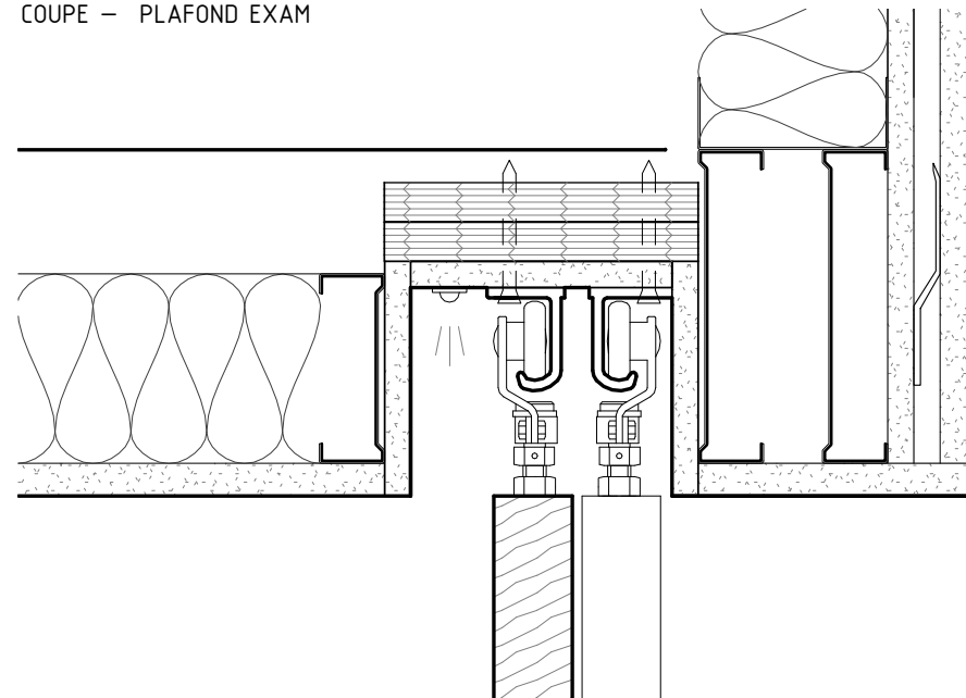
COUPE – COULISSE GARDE-ROBE
