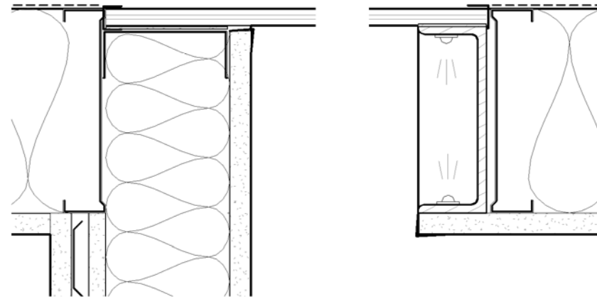
COUPE – PLAFOND EXAM
