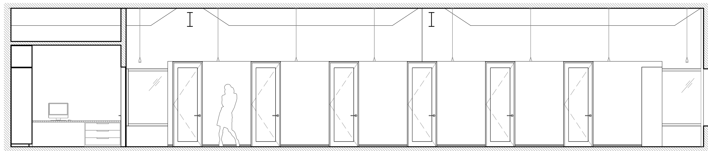
ÉLÉVATION INTÉRIEURE – SALLES D'EXAMEN
