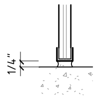
COUPE – VERRE / BÉTON
