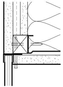
COUPE – VERRE / COIN GYPSE
