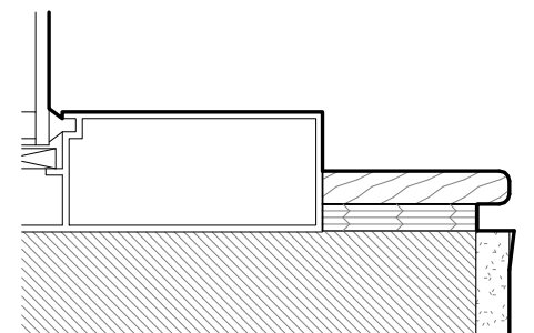
COUPE – ALLÈGE FENÊTRE
