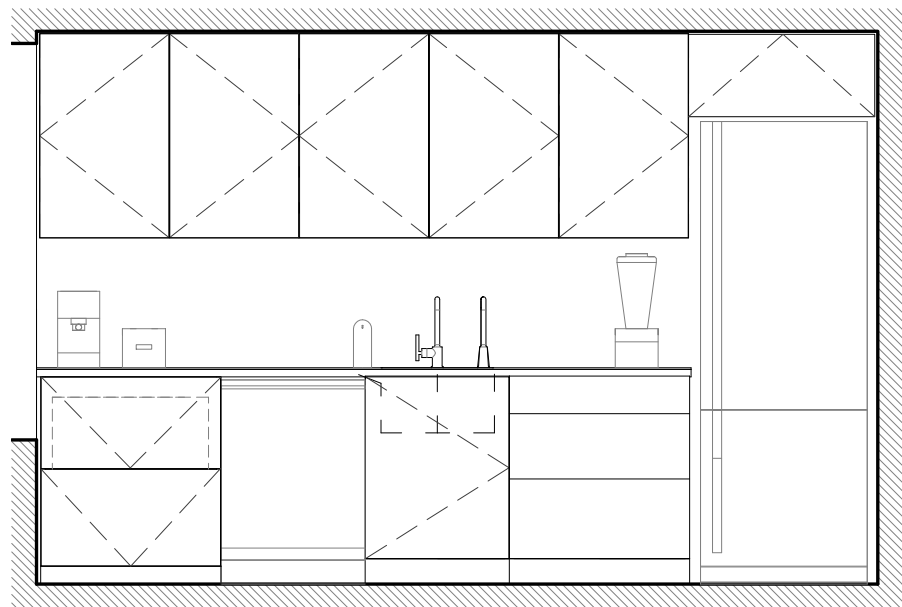
ÉLÉVATION – CUISINE
